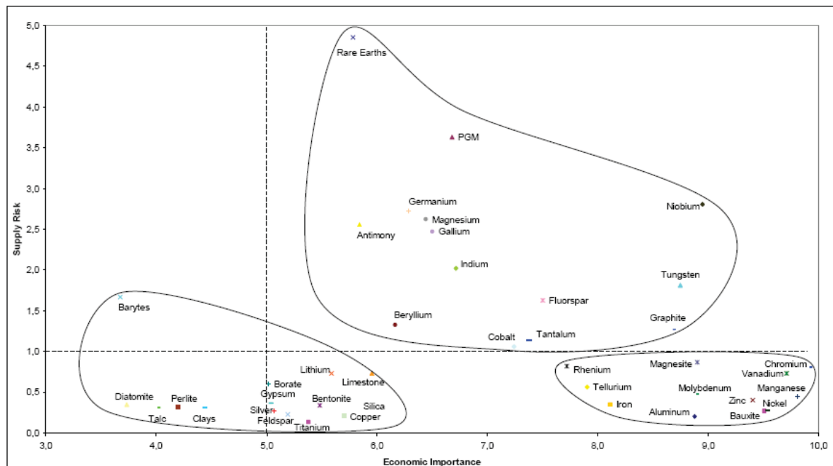
Abbildung 9: Clusterdarstellung des Rohstoffrisikos, Quelle: EU-Kommission (2010)
